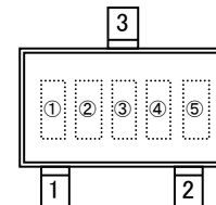
SOT-23(TO-236)
