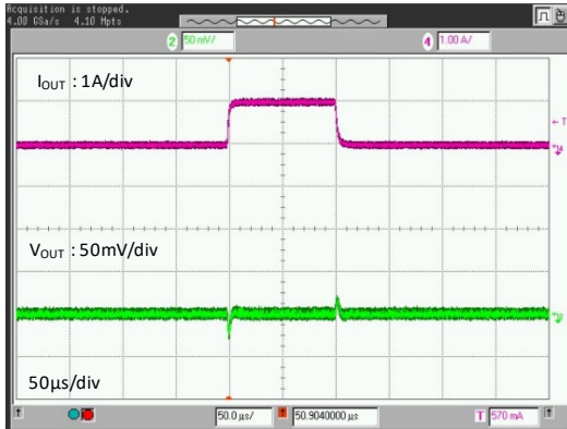
XCL237, V_{OUT(T)}=1.8V
