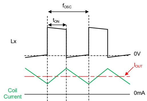
XCL238 シリーズ：重負荷動作例
