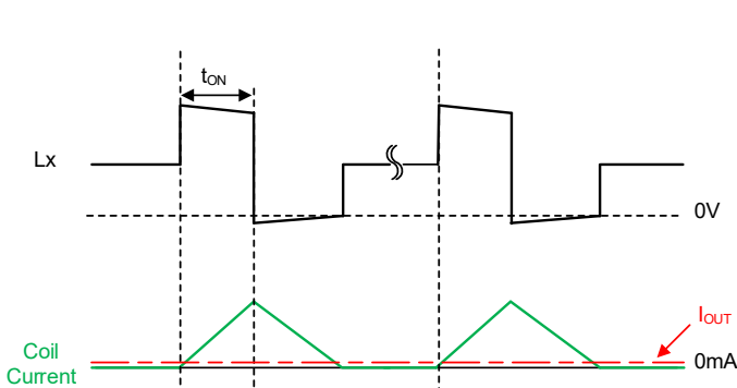
XCL238 シリーズ：軽負荷動作例
