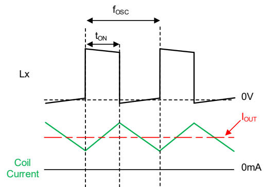
XCL237 シリーズ：重負荷動作例
