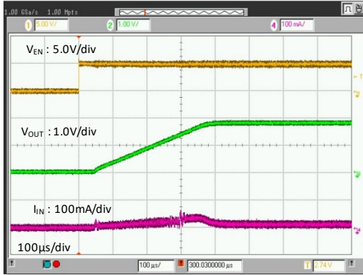
XCL237E, V_{OUT(T)}=1.8V
