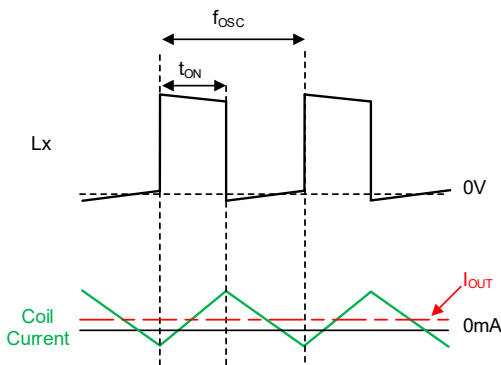
XCL237 シリーズ：軽負荷動作例
