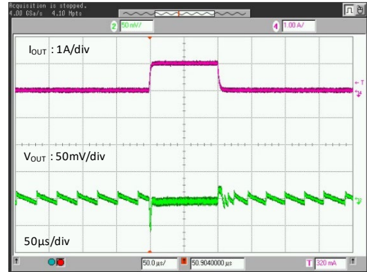
XCL238, V_{OUT(T)}=3.3V
