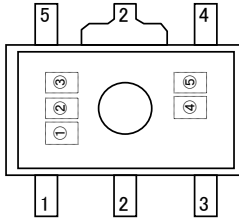
SOT-89-5
