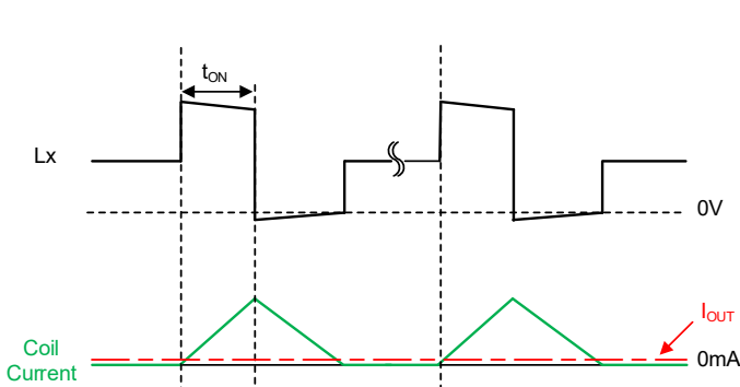
XC9288 シリーズ : 軽負荷動作例
