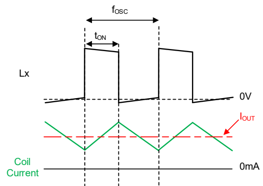
XC9287 シリーズ : 重負荷動作例
