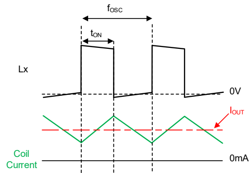
XC9288 シリーズ : 重負荷動作例
