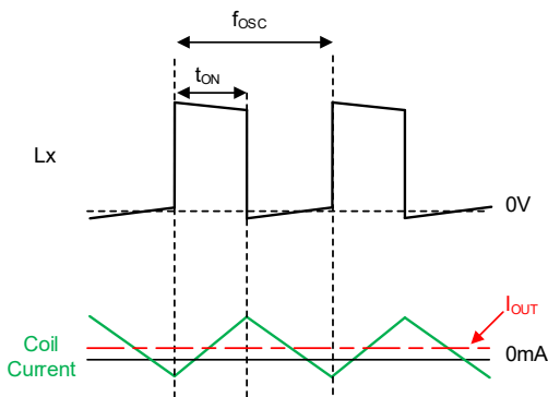
XC9287 シリーズ : 軽負荷動作例
