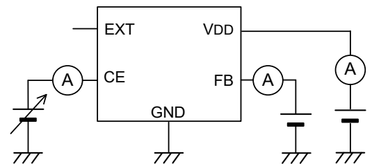
測定回路⑤
