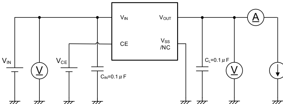
Test CIRCUITS④
