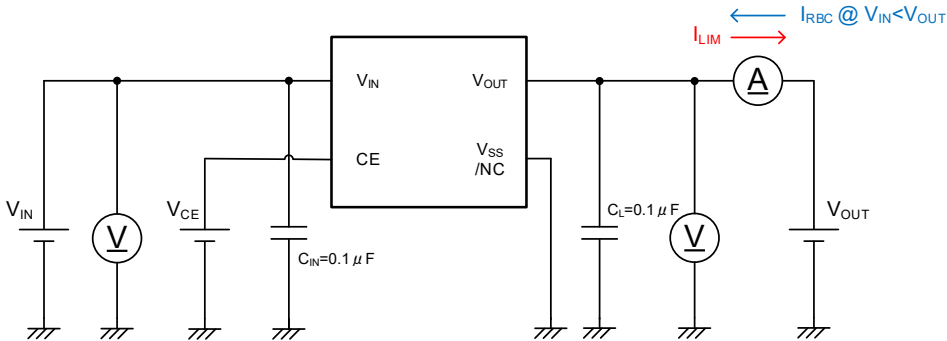
Test CIRCUITS③
