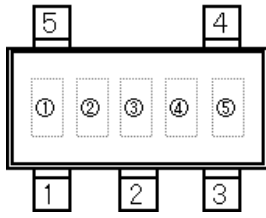
SOT-25
