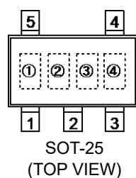
●SOT-25
