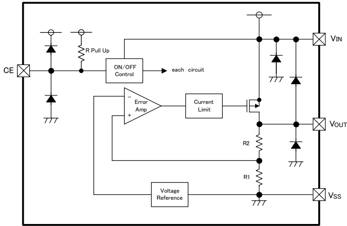
XC6219 シリーズ C/G タイプ
