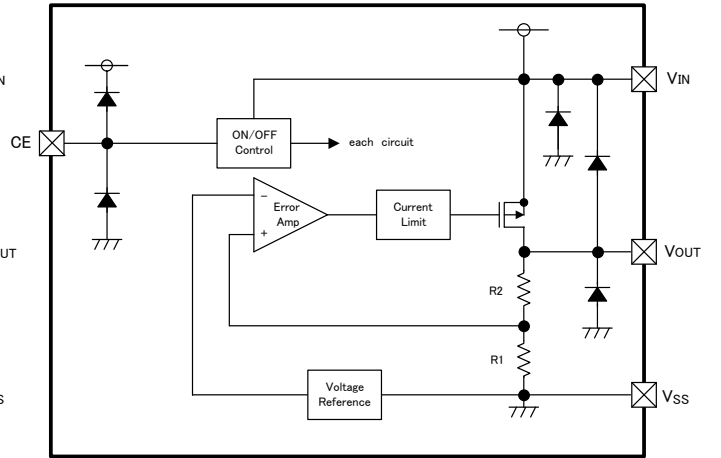
XC6219 シリーズ B/D/F/H タイプ
