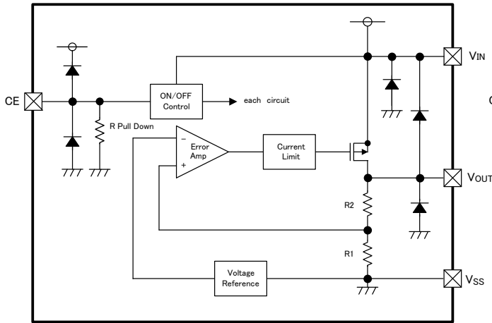
XC6219 シリーズ A/E タイプ
