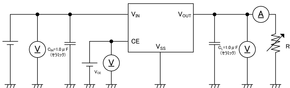
測定回路 1
