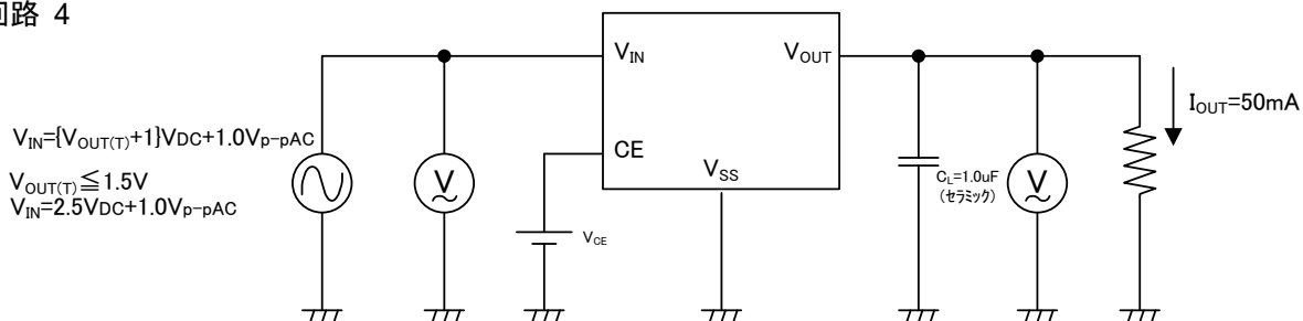
測定回路 4
