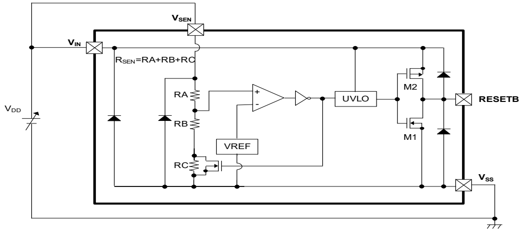
図 3：代表回路例 (CMOS 出力/Active Low 品)
