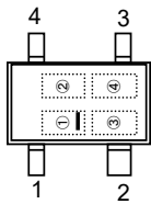
SSOT-24(マーク①下バー仕様)
