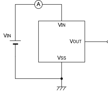
測定回路4
