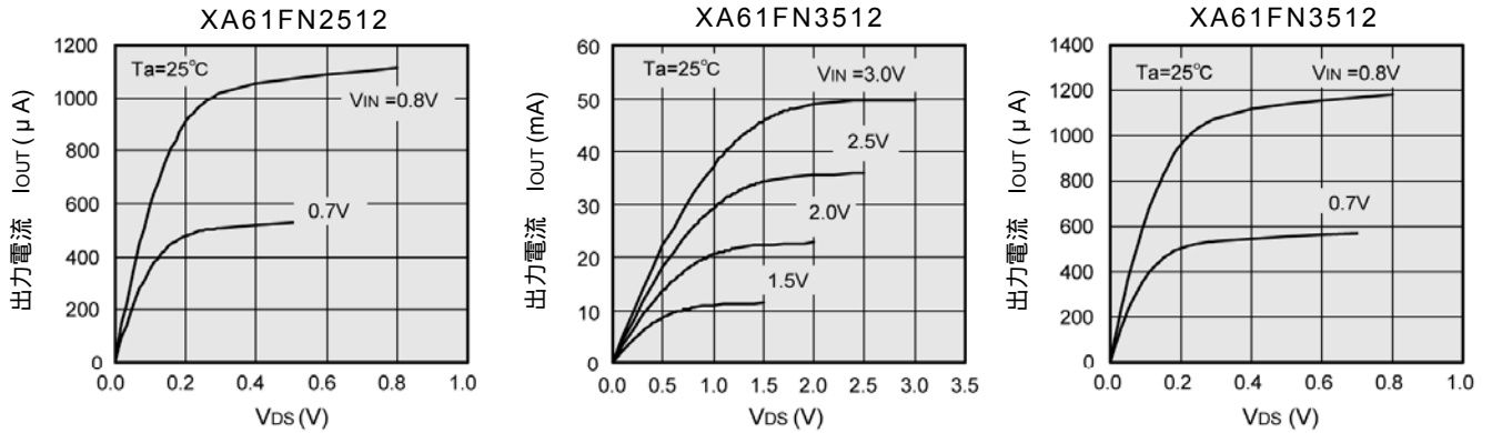
(4) Nch ドライバ出力電流 - V_{DS} 特性例
