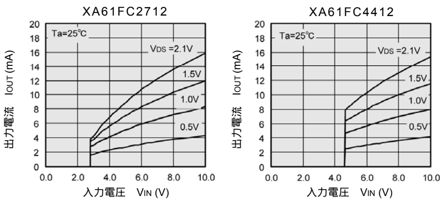
(6) Pch ドライバ出力電流 - 入力電圧特性例
