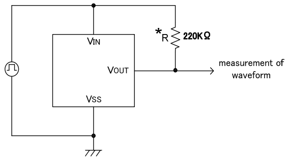
測定回路5
