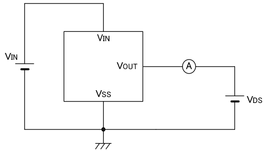
測定回路5
