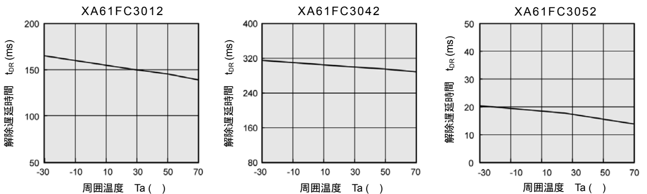
(7) 周囲温度 - 解除遅延時間 ( t_{DR} ) 特性例
