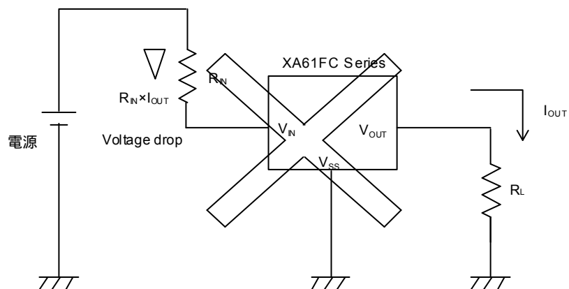
図 2 . 出力電流による発振
