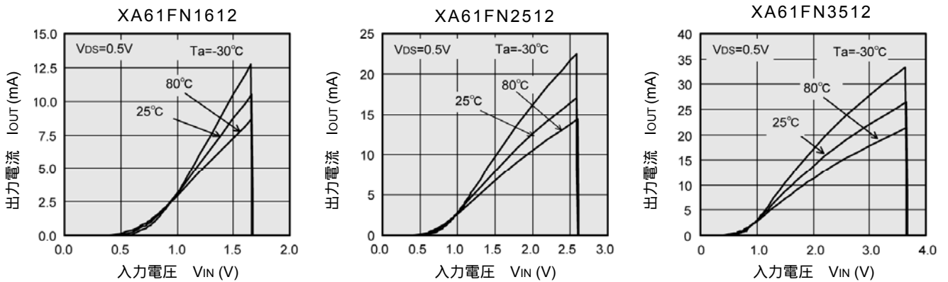
(5) Nch ドライバ出力電流 - 入力電圧特性例
